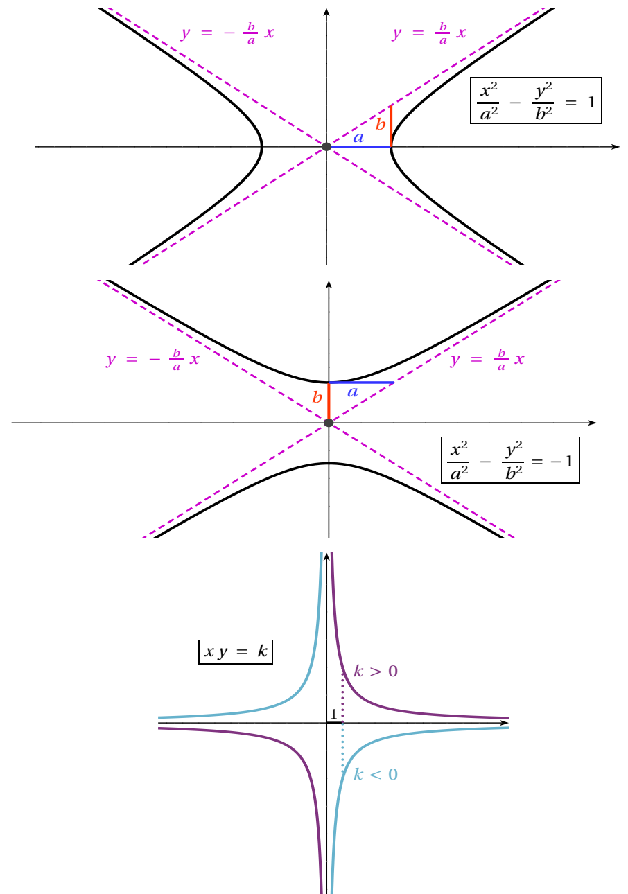
Hipèrbola
