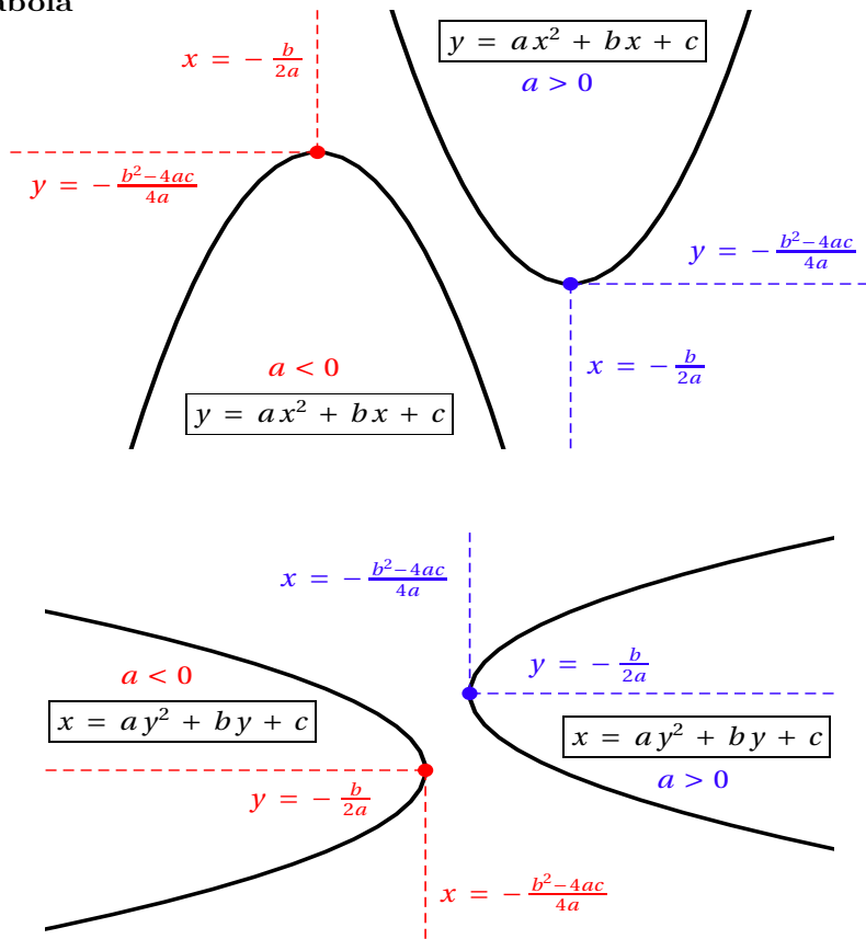
Paràbola
